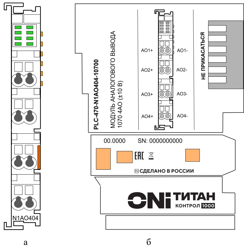
Рисунок 1 – Модуль N1AO404 (а – вид спереди, б – вид справа)
