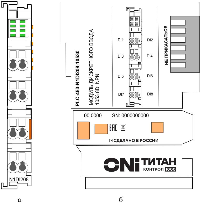
Рисунок 1 – Модуль N1DI208 (а – вид спереди, б – вид справа)
