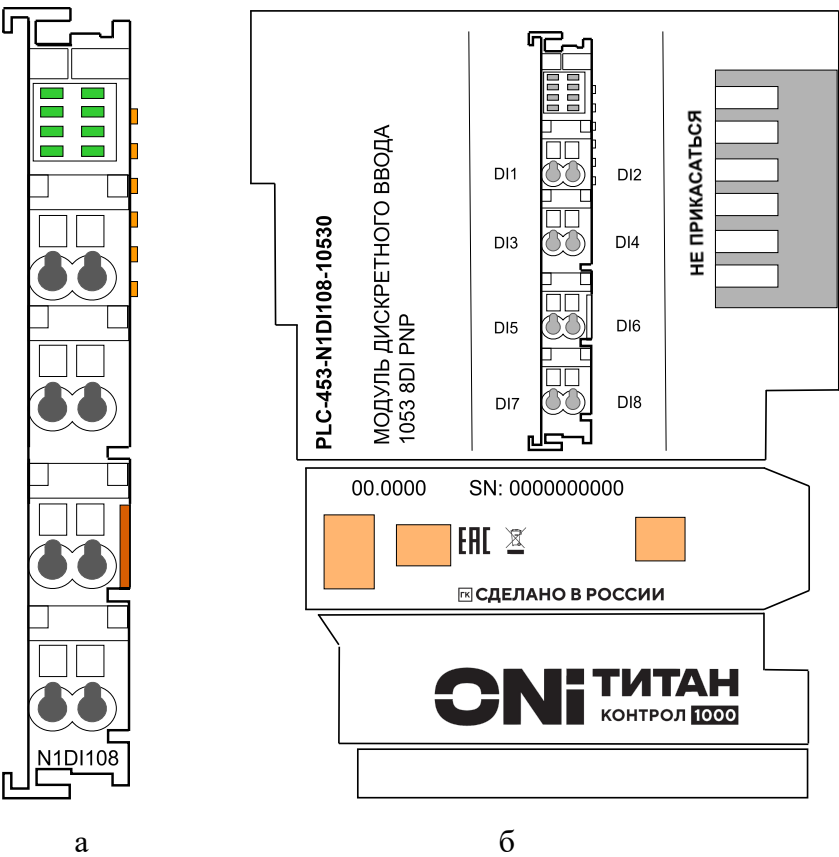
Рисунок 1 – Модуль N1DI108 (а – вид спереди, б – вид справа)
