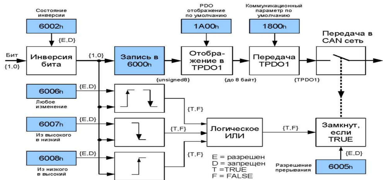
Рисунок 2 – Алгоритм работы модуля дискретного ввода
